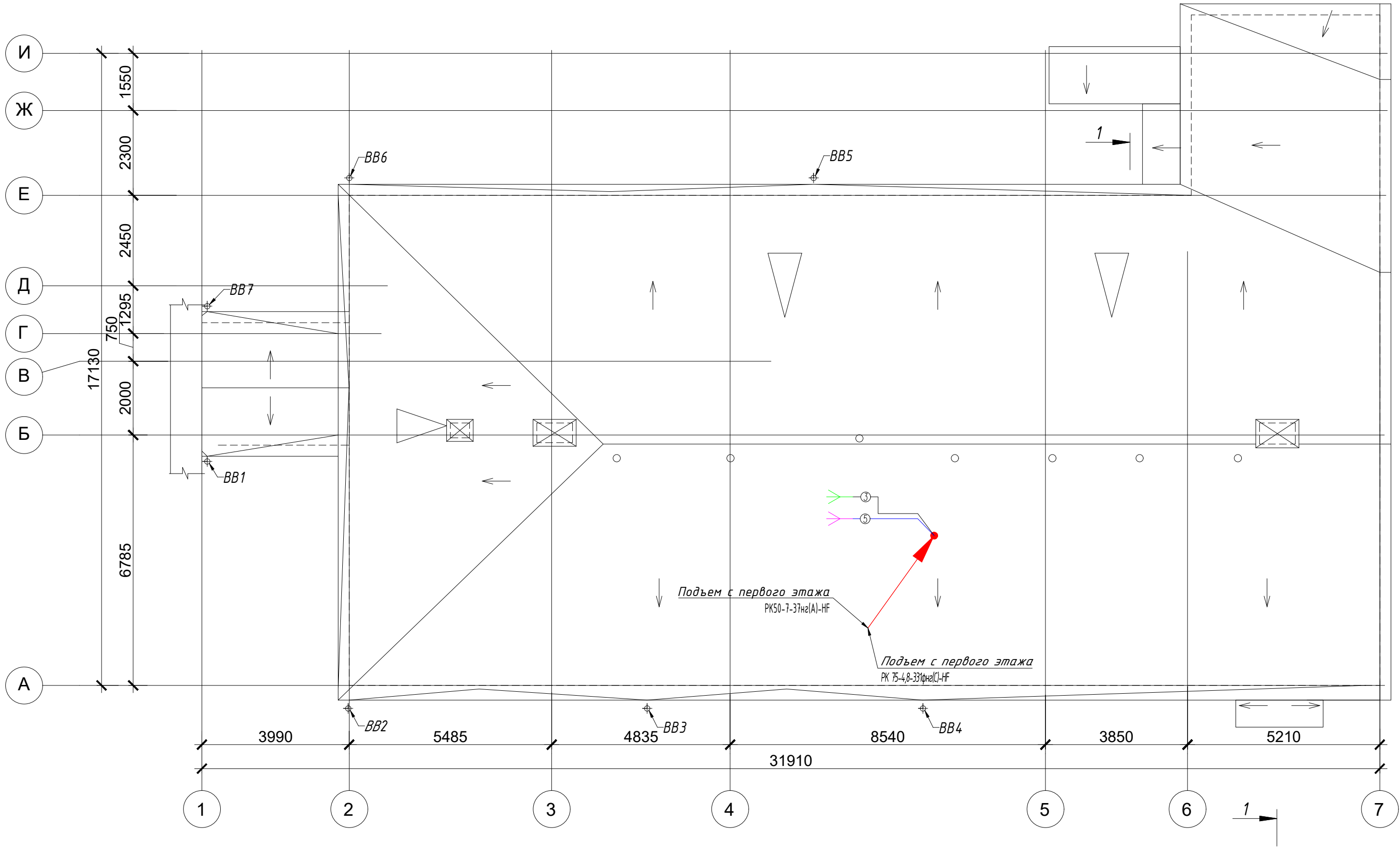
План кровли М 1:100
