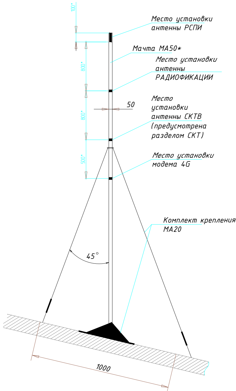
Эскиз крепления мачты на скатную кровлю
